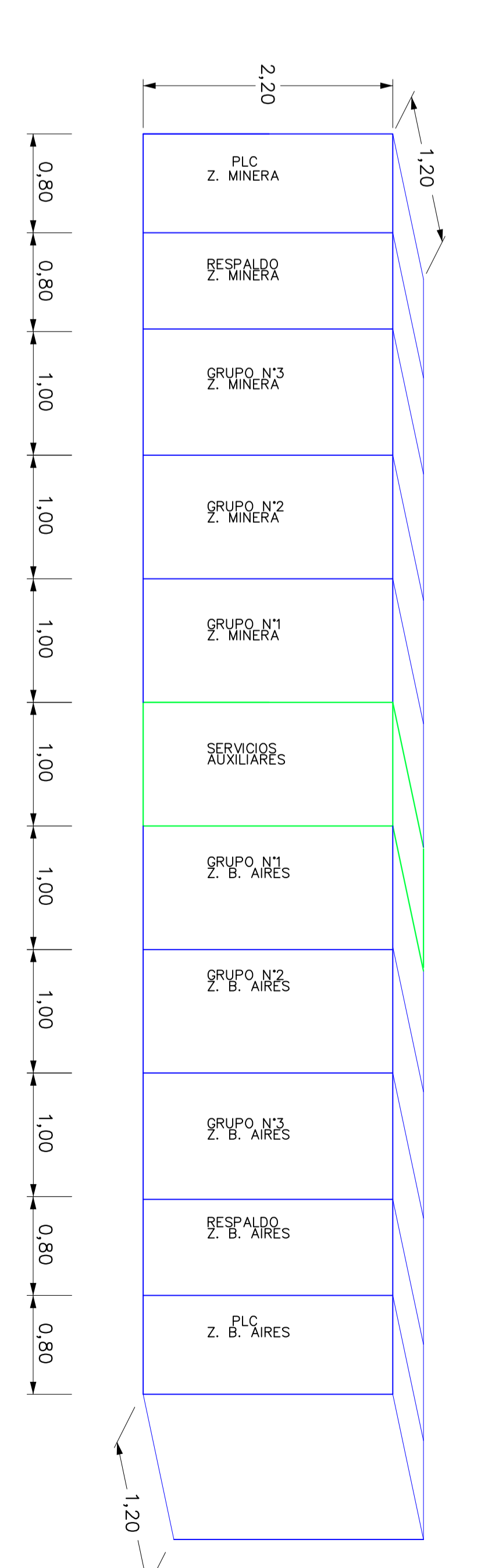
GRUPO MODULAR DE CELDAS ELÉCTRICAS Y CONTROL PARA LOS BOMBOS LA PLAYITA ZONA BUENOS AIRES Y ZONA MINERA VER DETALLE A
